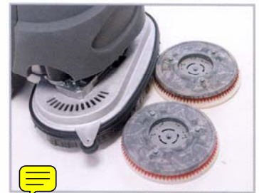
Changement des disques ou des brosses par un bouton placé sur la poignée des commandes pour augmenter la productivité.
